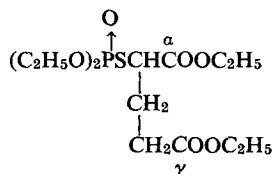
\alpha -Glutarate malaoxon
